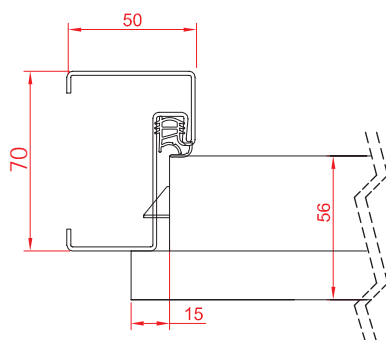
ajtótok
