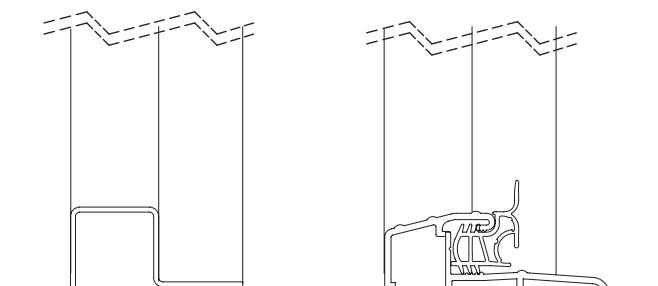
küszöb
