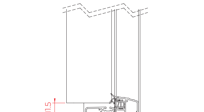
küszöb
